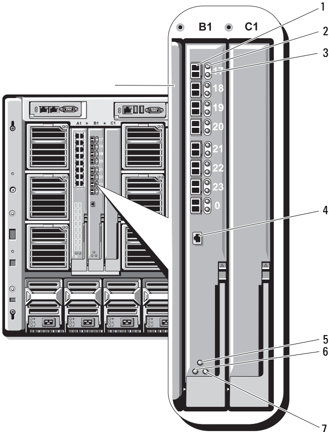
Figure 3-5. Caractéristiques du module d'E/S Brocade M4424 pour réseau SAN
